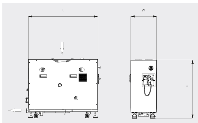
Dessin d'encombrement
