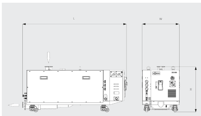
Disegno dimensionale
