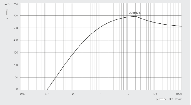
Saugvermögen
