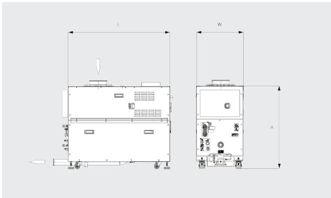
Maßblatt
