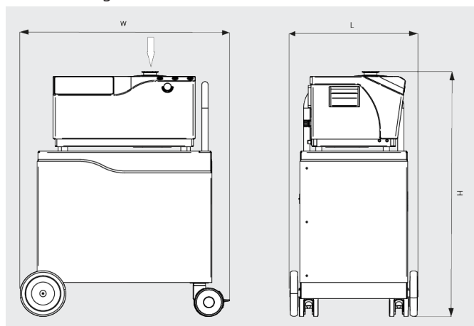
Maßzeichnung
