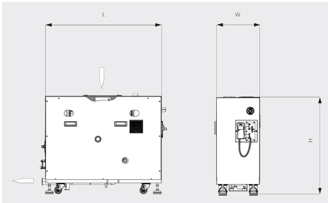
Maßzeichnung
