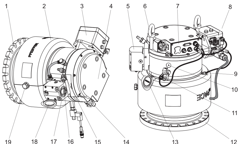
Fig. 2: HiPace 1200 T | UT design
