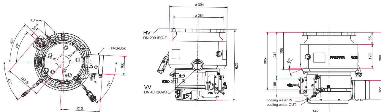
Fig. 36: HiPace 1200 T | TC 1200 DN 250 ISO-F
