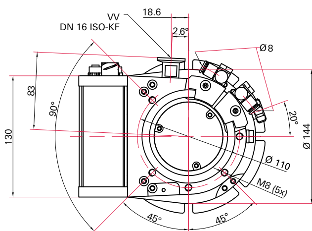
Fig. 16: HiPace 300 Plus, DN 100 ISO-F
